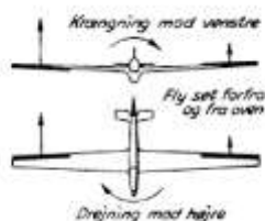
Krængerorenes sekundære virkning
